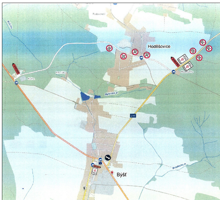
Objízdná trasa pro osobní automobily Dopravní opatření uzavírka I/35 - Býšť – „detail 4“
